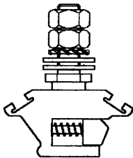
Monoborne MH-6 fabricado en resina poliester y bronce niquelado
