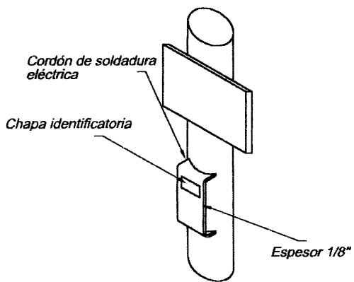
DETALLE CHAPA SOSTEN DE CAJA Y PLACA
